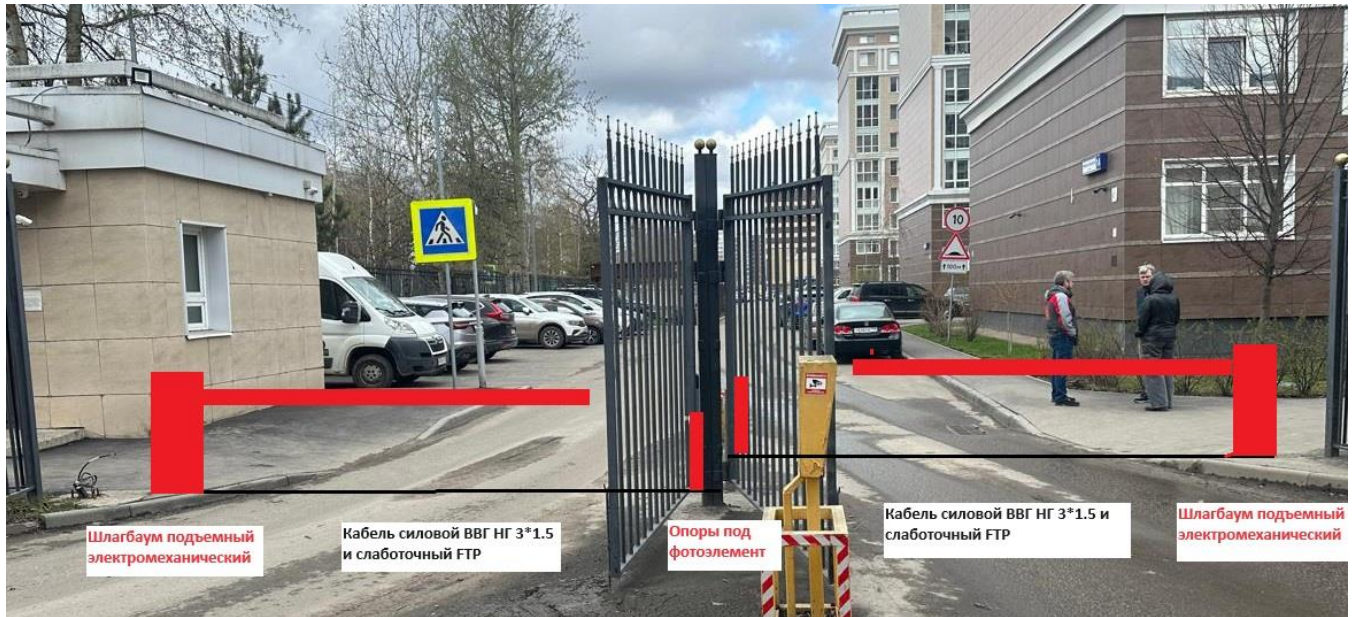
Рис. 1 Схема размещения шлагбаумов
