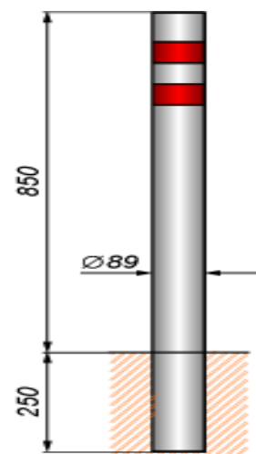
Рис. 4. Внешний вид и размеры столбика заграждения
